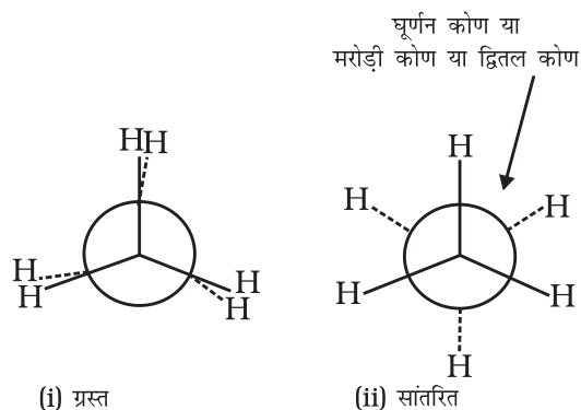
चित्र 9.3 एथेन के न्यूमैन प्रक्षेप
