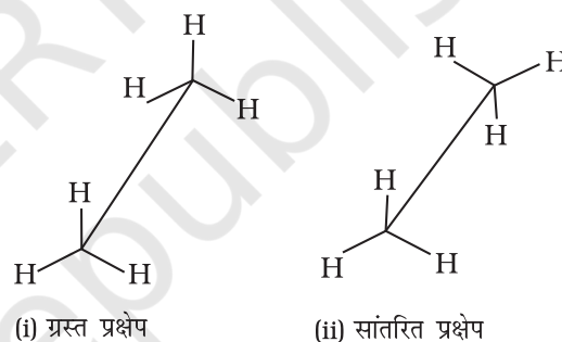
चित्र 9.2 एथेन के साहार्स प्रक्षेप
