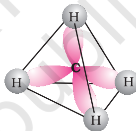
चित्र 9.1 मथेन ( \text{CH}_4 ) की चतुष्फलक संरचना
