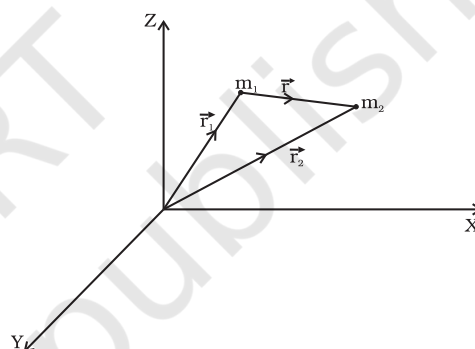
चित्र 7.3 m_2 के कारण m_1 पर गुरुत्वीय बल \mathbf{r} के अनुदिश है, यहाँ \mathbf{r}, (\mathbf{r}_2 - \mathbf{r}_1) है।
