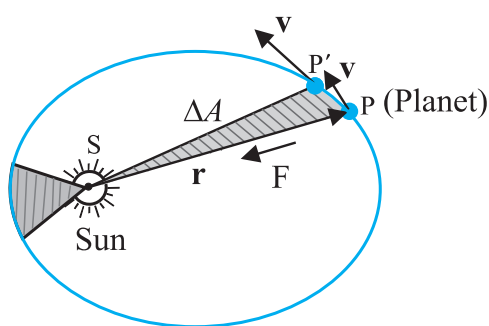
चित्र 7.2 ग्रह P सूर्य के परितः दीर्घवृत्तीय कक्षा में गति करता है। किसी छोटे समय अंतराल \Delta t में ग्रह द्वारा प्रसरित क्षेत्रफल \Delta A को छायांकित क्षेत्र द्वारा दर्शाया गया है।
