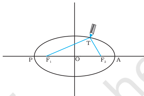
चित्र 7.1(b) एक दीर्घवृत्त खींचना। एक डोरी के दो सिरे F_1 तथा F_2 स्थिर हैं। पेंसिल की नोक डोरी को तनी रखते हुए इन सिरों के परितः चलायी जाती है।
