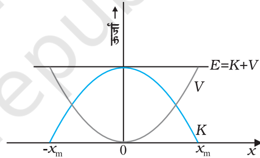
चित्र 5.8 किसी स्प्रिंग से जुड़े हुए गुटके की स्थितिज ऊर्जा V और गतिज ऊर्जा K के परवल्यिक आलेख जो हुक के नियम का पालन करते हैं। ये एक-दूसरे के पूरक हैं अर्थात् इनमें जब एक घटता है तो दूसरा बढ़ता है, परंतु कुल यांत्रिक ऊर्जा E = K + V हमेशा अचर रहती है।
