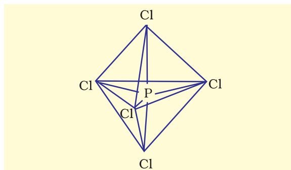
चित्र 4.17 PCl_5 अणु की त्रिकोणीय द्वि-पिरामिडी ज्यामिति
