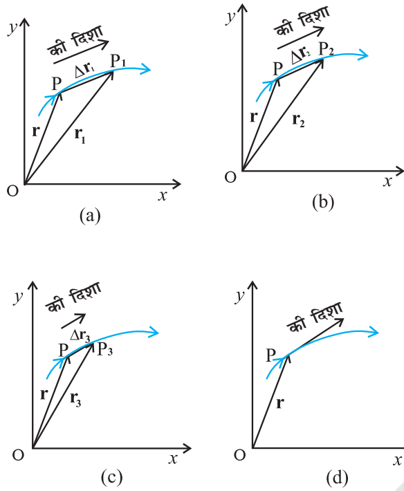
चित्र 3.13 जैसे ही समय अंतराल \Delta t शून्य की सीमा को स्पर्श कर लेता है, औसत वेग \bar{\mathbf{v}} वस्तु के वेग \mathbf{v} के बराबर हो जाता है। \mathbf{v} की दिशा किसी क्षण पथ पर स्पर्श रेखा के समान्तर है।
