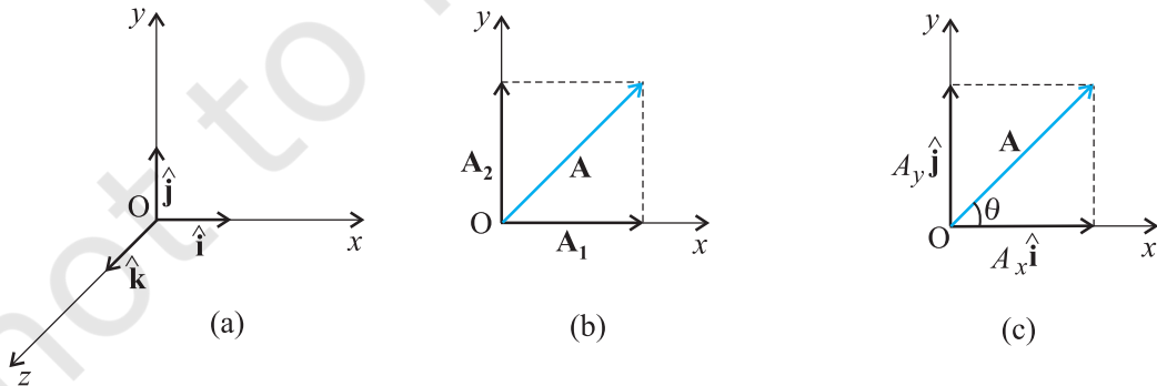
चित्र 3.9 (a) एकांक सदिश \hat{i}, \hat{j}, \hat{k} अक्षों x, y, z के अनुदिश हैं, (b) किसी सदिश \mathbf{A} को x एवं y अक्षों के अनुदिश घटकों \mathbf{A}_1 तथा \mathbf{A}_2 में वियोजित किया है, (c) A_x तथा A_y को \hat{i} तथा \hat{j} के पदों में व्यक्त किया है।
