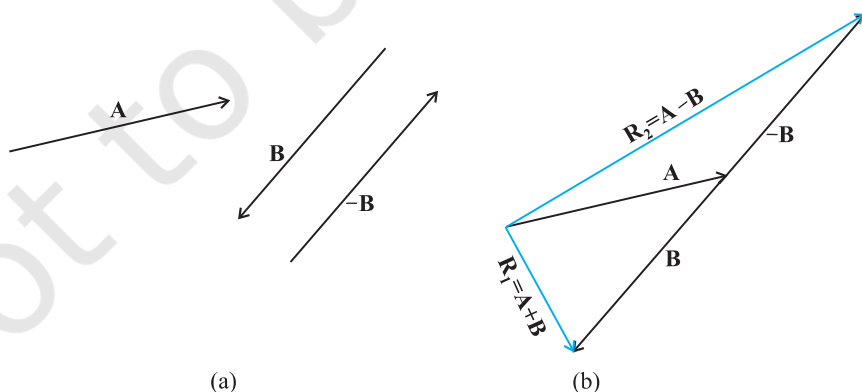
चित्र 3.5 (a) दो सदिश A व B , -B को भी दिखाया गया है। (b) सदिश A से सदिश B का घटाना-परिणाम R 2 है। तुलना के लिए सदिशों A व B का योग R 1 भी दिखाया गया है।
