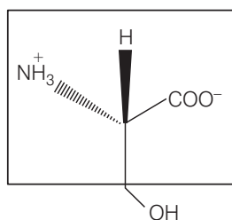
L-serine
