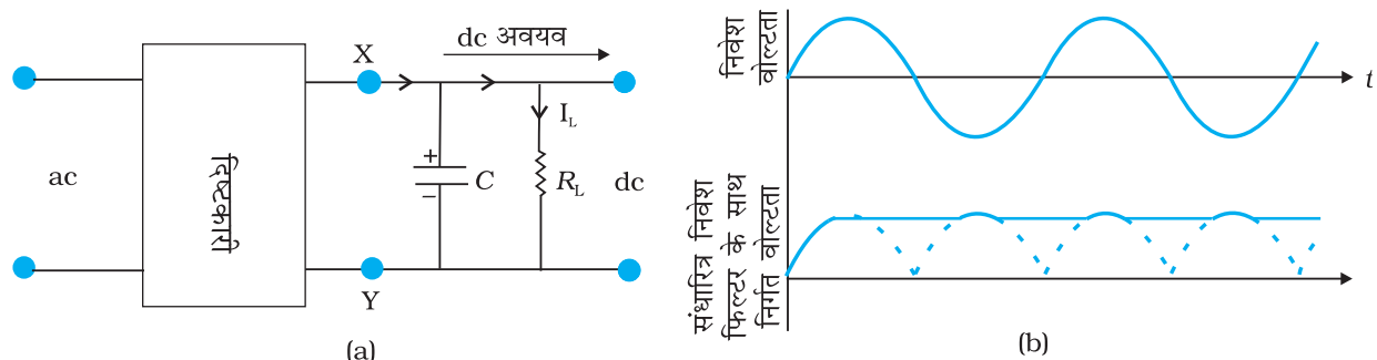
चित्र 14.20 (a) संधारित्र फिल्टर के साथ पूर्ण तरंग दिष्टकारी, (b) में दिष्टकारी की निवेश तथा निगत वोल्टता।
